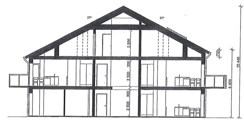
SEKTION B-B 1:100
