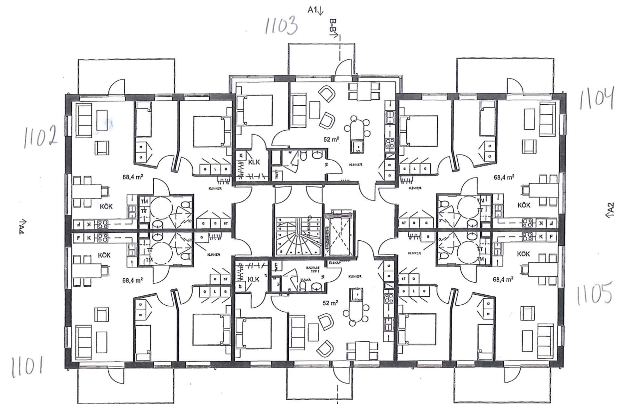
PLAN 2 1:100
