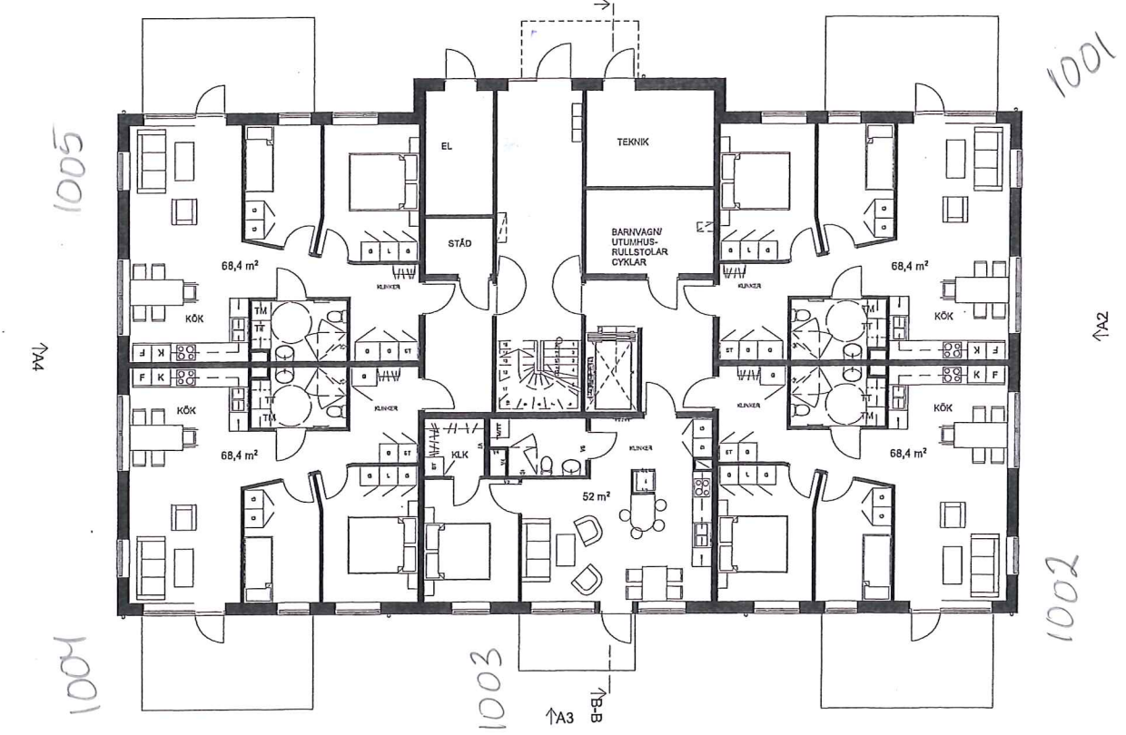
PLAN 1 1:100
