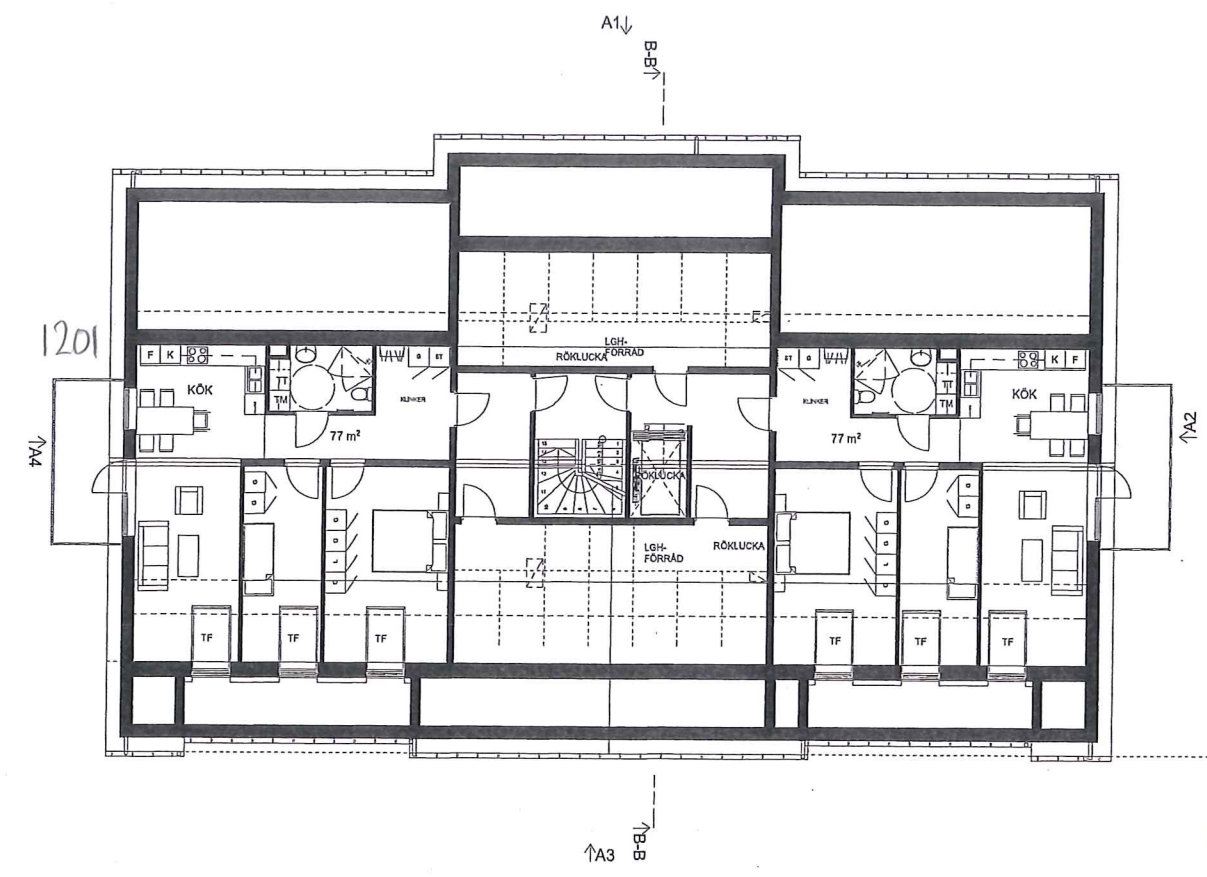
VINDSPLAN 1:100
